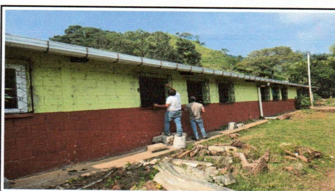
Foto 4: Cambio de ventana de metal a pvc por deterioro y seguridad de la escuela.
