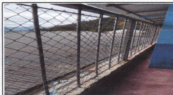
Foto 5: sustitucion de tubos AG. De 1 pulgada en malla
