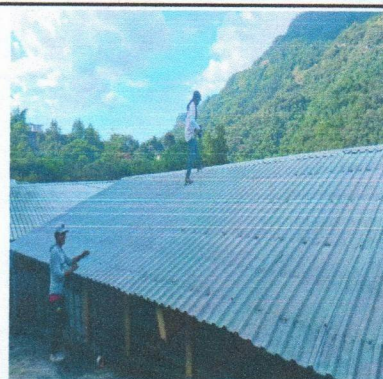
Foto 8: CUBIERTA DE LAMINA Sustitución de lámina, por lámina troquelada aluzinc calibre 26
