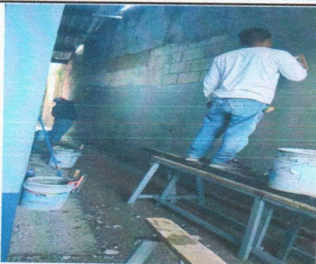
Foto1: REPARACION DE REPELLO Y CERNIDO DE PAREDES (CUANDO APLIQUE) reparación de repello y cernido de paredes
