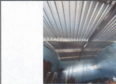
Foto1: Sustitucion de lamina, por lamina troquelada calibre 26
