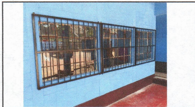
Foto 4: Sustitucion de balcones de metal de 2.30 mts. Por 1.30 mts y 1.35 mts. Por 1.20 mts.
