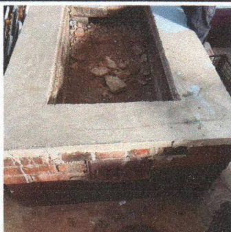
Foto 5: Sustitución de plancha de tres hornillas de cocina
