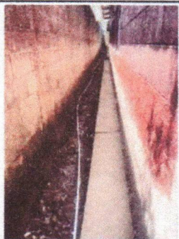
Foto 3: Reparación de cuneta de cemento
