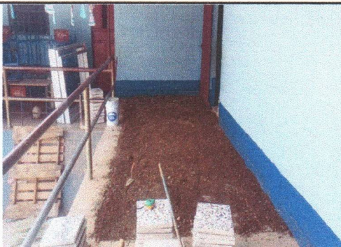
Foto1: Sustrución de piso de concreto por piso tipo granito
