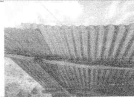
FOTO 6: Sustitución de estructura de madera por estructura de metal
