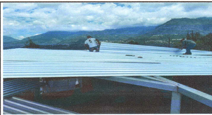
Foto 4: Sustitución de lámina por lámina troquelada aluzinc calibre 26 en modulo 4
