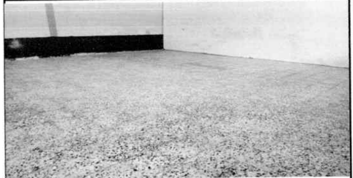
Foto 2: Colocación de piso de granito
