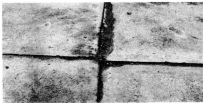
Foto 6: Sustitución de plancha de concreto
