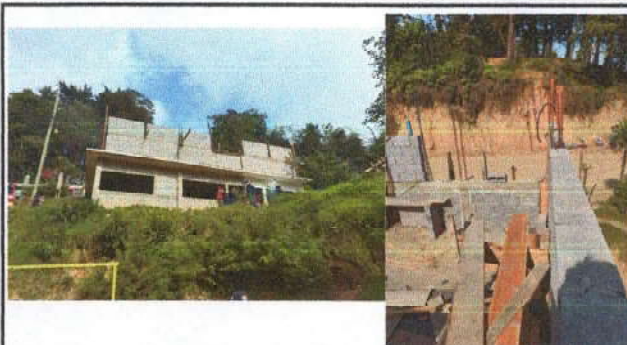
Foto 9: Mejoramiento a estructura de soporte de metal
