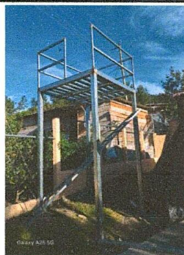
Foto 2: estructura de metal para la ubicación de depósito de agua
