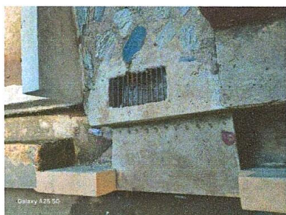
Foto 3: reparacion de cuneta para el desplazamiento de agua pluvial
