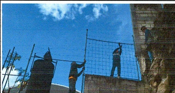
Foto 3: 9.1 Sustitución de malla galvanizada por electromalla
