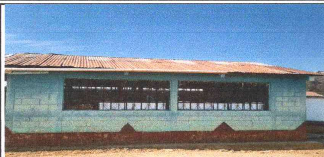
FOTO 1. SUSTITUCION DE LAMINA, POR LAMINA TROQUELADA ALUZINC CALIBRE 26
