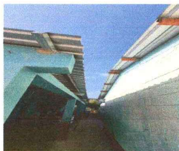
Foto 6: SUSTITUCIÓN DE CANAL DE METAL, CON SOPORTE, TAPONES Y BAJADAS.
