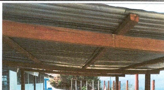
Foto 1: sustitución de techo de lámina, por lámina troquelada calibre 26
