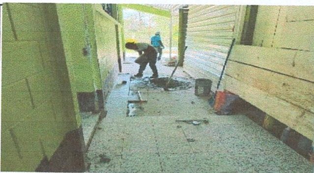
Foto 3: Proceso de instalación de piso de granito en patio
