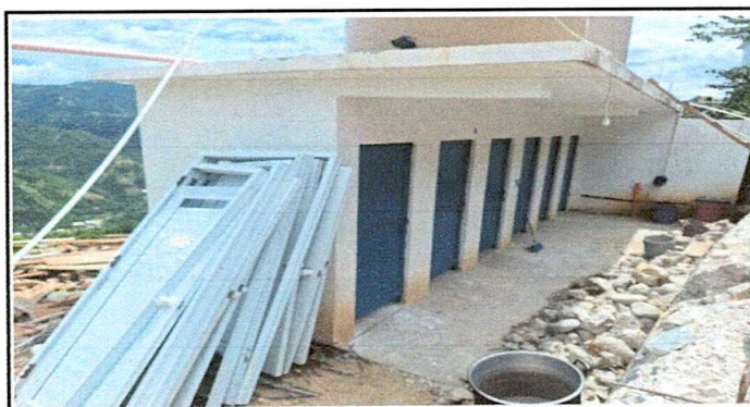
Foto 3: Instalación de 6 puertas para baño
