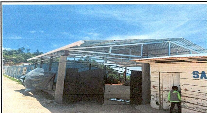
Foto1: Instalación de bajadas de agua
