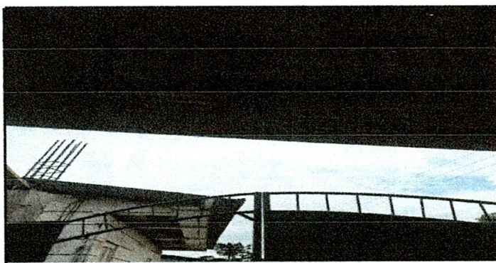
Foto 5: Lámina de techo en mal estado, se pueden observar perforaciones de la lámina
