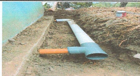
Foto 14: Proceso de mantenimiento de drenaje de sanitarios
