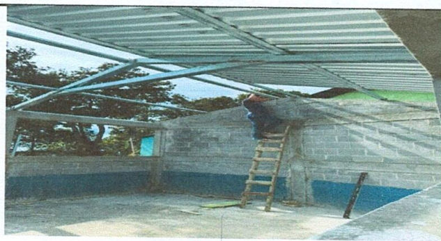
Foto 9: Proceso de mejoramiento de techo de aula ya que carece del mismo por ser aula nueva.
