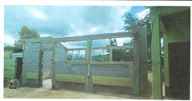
Foto 20: Mejoramiento de ventana de aula ya que carece de la misma, parte de enfrente.
