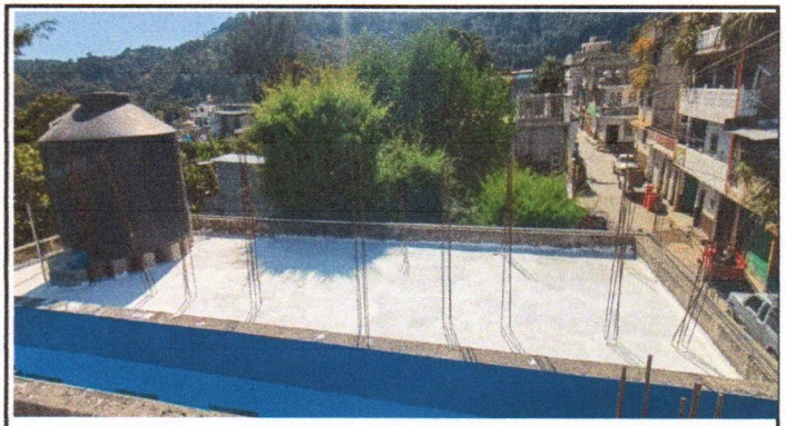
Foto 4: IMPERMEABILIZACIÓN DE LOSA
