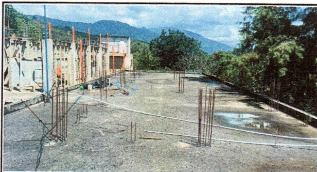
Foto 3: IMPERMEABILIZACIÓN DE LOSA
