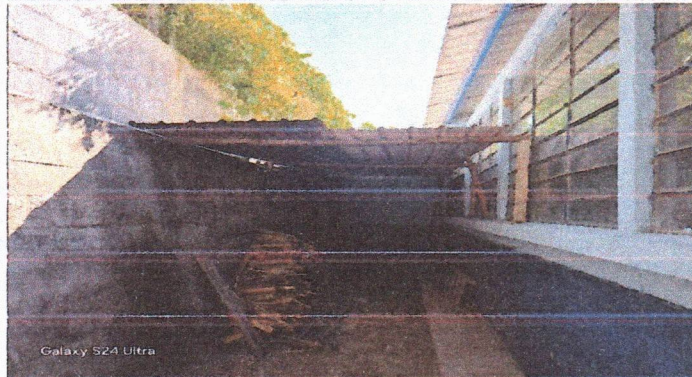
Foto 1: Sustitución de estructura de madera por costanera galvanizada chapa 14 original
