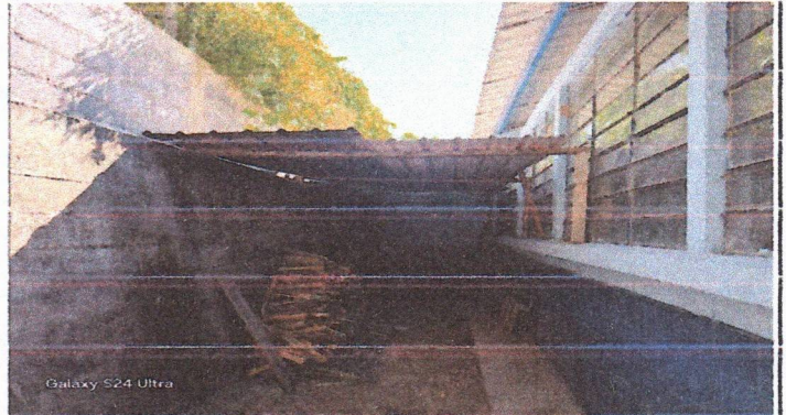
Foto 2: Sustitución de lámina por lámina troquelada calibre 24
