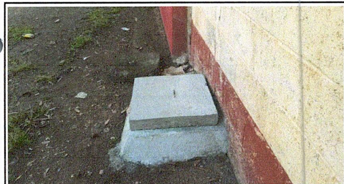
Foto 9: CAJA REPOSADERA DE DESHECHOS CONSTRUIDA Y FINALIZADA.
