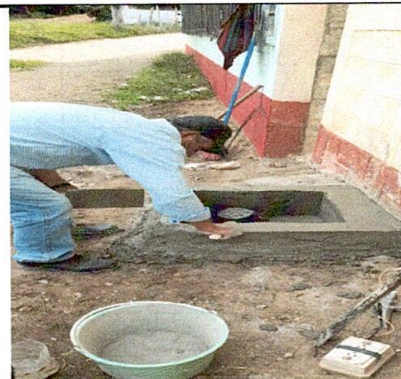
Foto 10: CONSTRUCCION DE CAJA REPOSADERA
