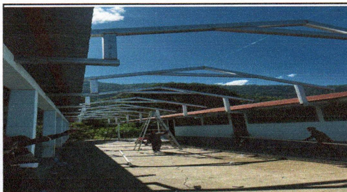
Foto 3: Sustitución de soporte de madera, por metal
