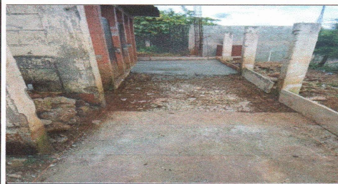
Foto 5: Sustrucción de piso de torta de concreto
