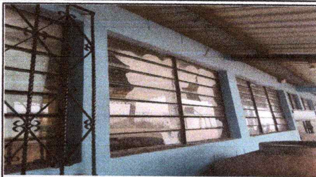
Foto 2: Mejoramiento de balcones de metal
