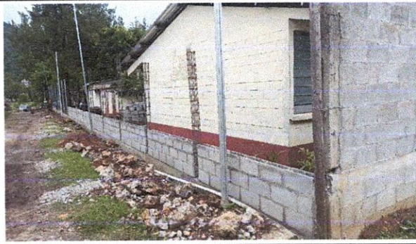
Foto 6: Mejoramiento de circulación perimetral en proceso.
