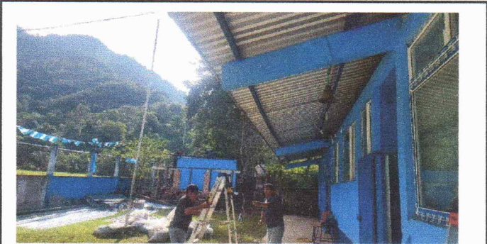
Foto 10: sustitución de canal con sus accesorios
