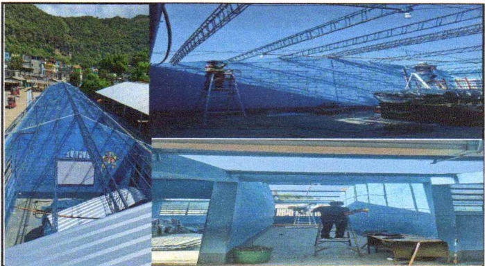
Foto 4: Mantenimineto a estructura de soporte de metal
