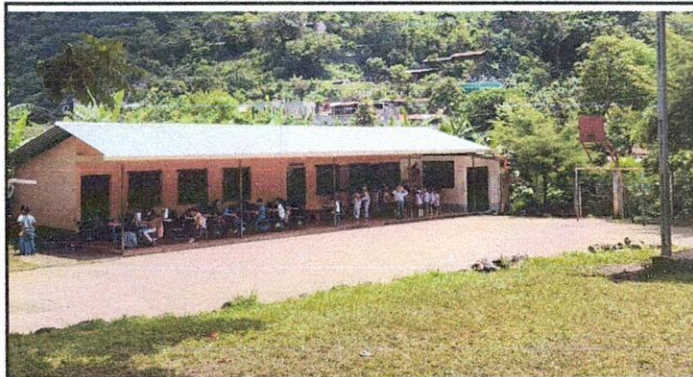
Foto 1: Lámina nueva, colocación nueva de soporte de metal, canal pluvial y bajada de agua.
