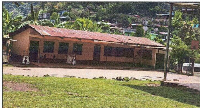
Foto 1: Lámina, soporte de madera, canal pluvial y bajada de agua en malas condiciones.
