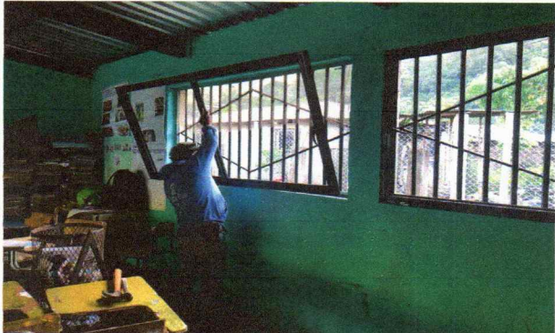
Foto 2: Mejoramiento de estructura de metal de ventana de 2.00 mts. de largo por 1.00 mt. de ancho.
