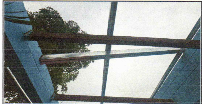
Foto 5: Estructura de techo de madera en proceso de descomposición.
