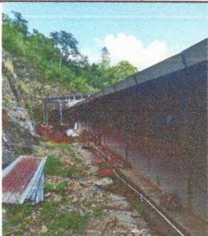
Foto 4: En esta imagen se evidencia la correcta instalación del nuevo canal de metal, con un acabado uniforme y asegurado a la estructura. La sustitución garantiza mayor durabilidad, resistencia y un mejor funcionamiento del sistema de drenaje pluvial.
