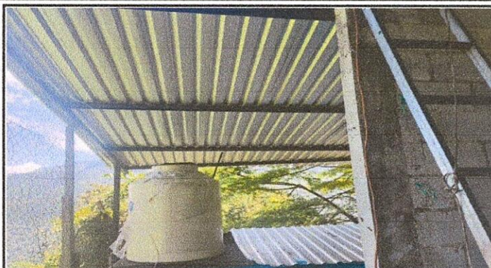
Foto 1: Cambio de techo de lámina por lámina troquelada calibre 26
