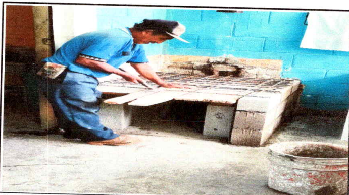
Foto 4: Cambio de estufa rural (completa) incluye chimeneas de cemento y plancha grande de metal.
