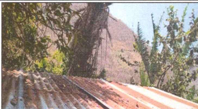
Foto 1: Lamina deteriorada
