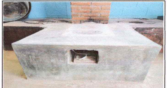
Foto 10: Mantenimiento de estufa rural.
