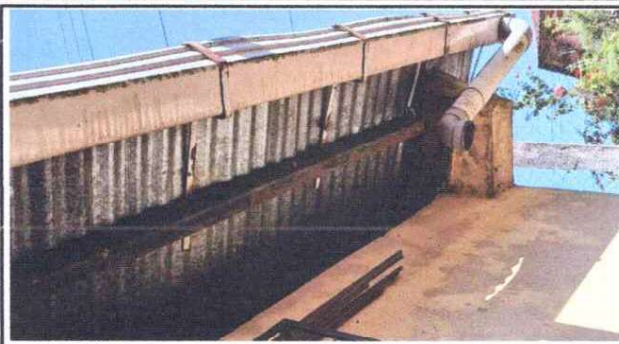
Foto 2: Estructura metálica oxidada de las aulas, desalineada, debido a la filtración del agua provocó el deterioro del material.
