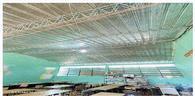
Foto 2: Sustitucion de estructura metalica
