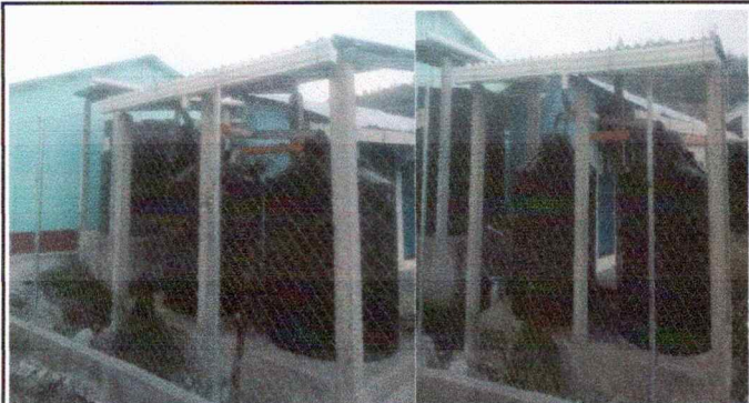
Foto 7: Mejoramiento de canal de pvc y bajada de agua pluvial, tubo PVC 3"
