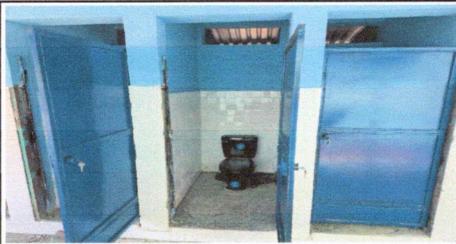
Foto 3: Mantenimiento a estructura (lijado, ampliación, aplicación de pintura y colocación de chapa) de 0.81 centímetros de ancho por 1.80 metros de alto
