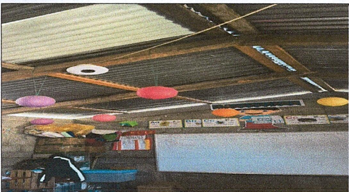
foto3: cambio de soporte de madera por metal
