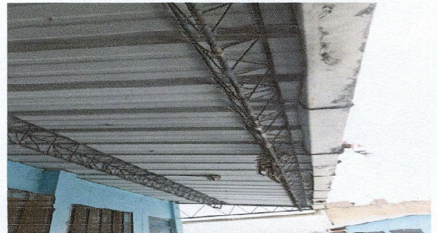
Foto 10: MEJORAMIENTO Y SUSTITUCIÓN DE CANALES PLUVIALES
