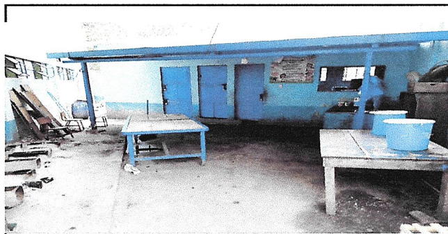
Foto 6: Construcción de 3 mesones de concreto para preparar los alimentos de 2.50 de largo x 0.60 de ancho x 0.90 de altura.
