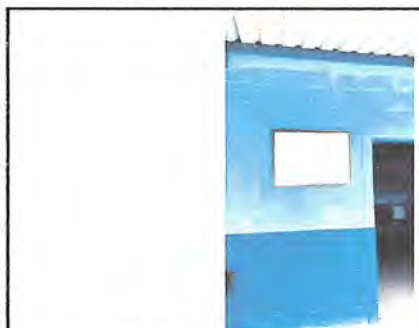
Foto 3: IMPLMENTACION DE VENTANA EN PARED FRONTAL EN AREA DE COCINA DE 1.20MTS DE ANCHO X 1.00 MT DE ALTURA, CON BALCON METALICO RETICULADO.
