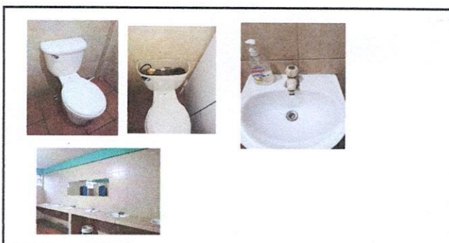
Foto 6: sustitucion de sanitarios y lavamanos con sus accesorios
