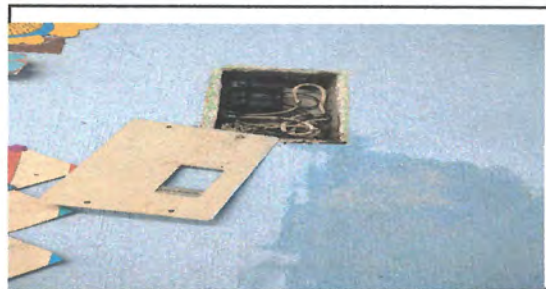
Foto 19: SUSTITUCION DE TUBERIA EN CAJA TIPO OCTAGONAL Y CABLEADO
