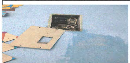
Foto 21: SUSTITUCION DE TABLERO DE 4 A 8 CIRCUITOS INCLUYE SU INSTALACION Y CONEXION DE CIRCUITOS
